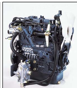
エンジン
