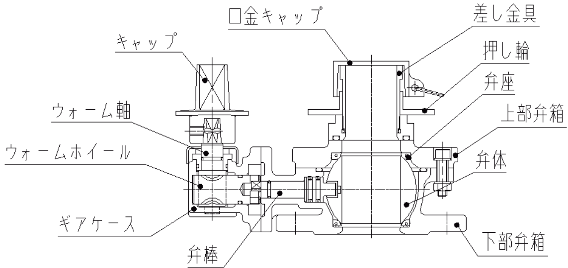
図 1 構造図
