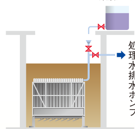
薬液タンク
