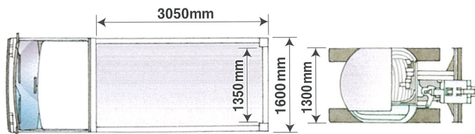
2t三転ダンプとのサイズ比較
