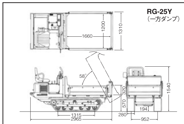
■ RG-25Y 寸法図
