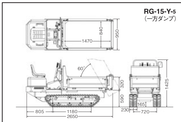
■ RG-15-Y-5 寸法図
