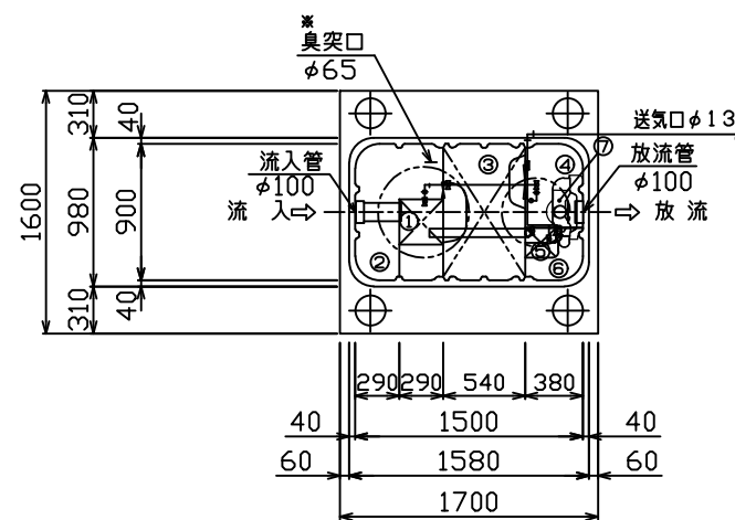
平面図 S=1/40
