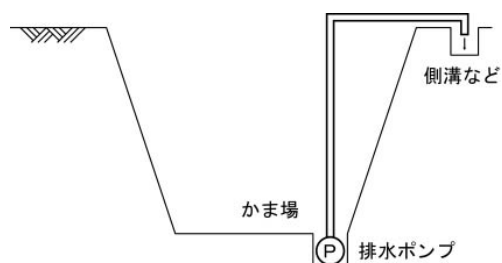
図 3 水替え工法
