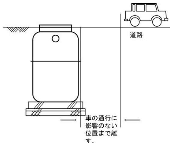
図 7 道路際から離して設置する例
