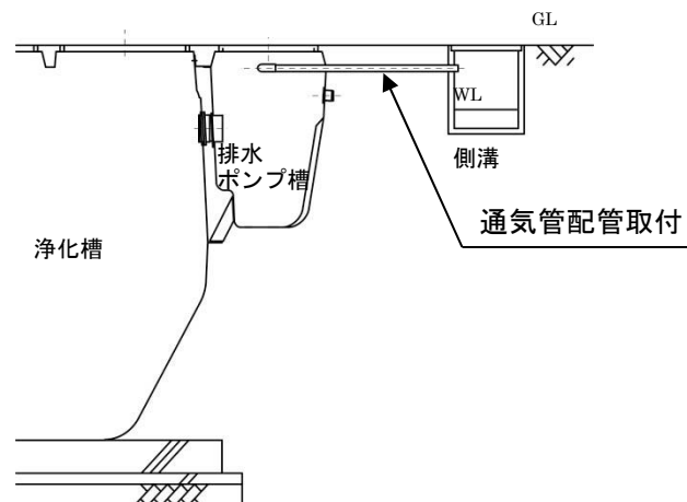
図14 通気配管の取付例
