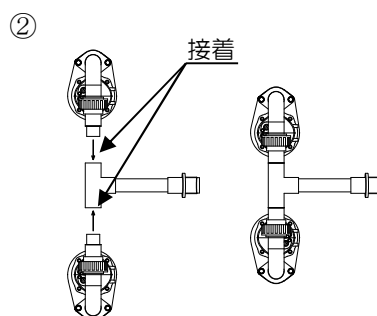
図13 配管方法取付図（平面）
