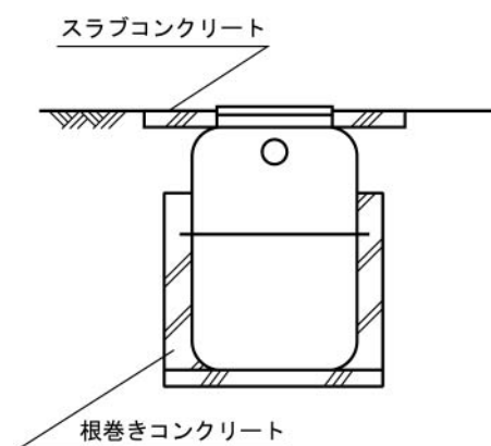
図 4 根巻きコンクリートの例
