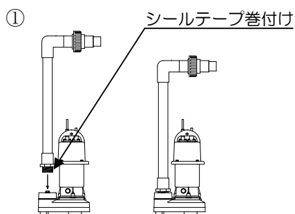
図12 配管方法取付図（断面）
