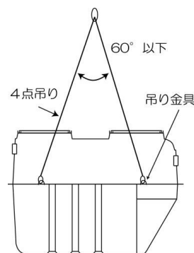
ワイヤーロープのかけ方
