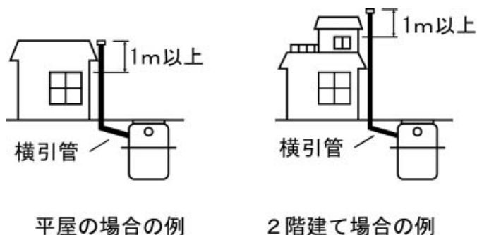
図9 臭突の設置例
