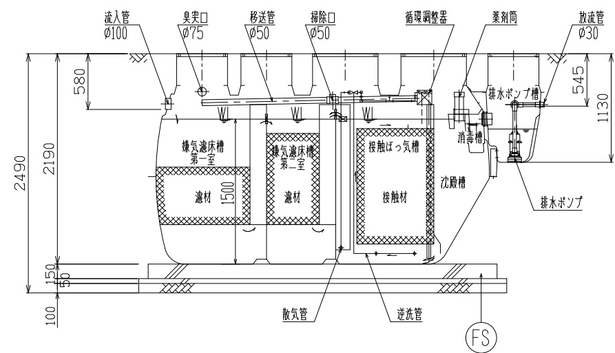
断面図 S=1/40
