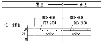
スラブ断面リスト S=1/40
