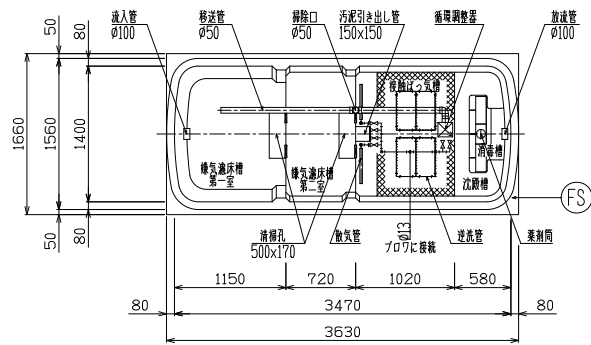
平面図 S=1/40
