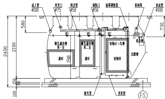
断面図 S=1/40
