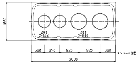
スラブ平面図 S=1/40
