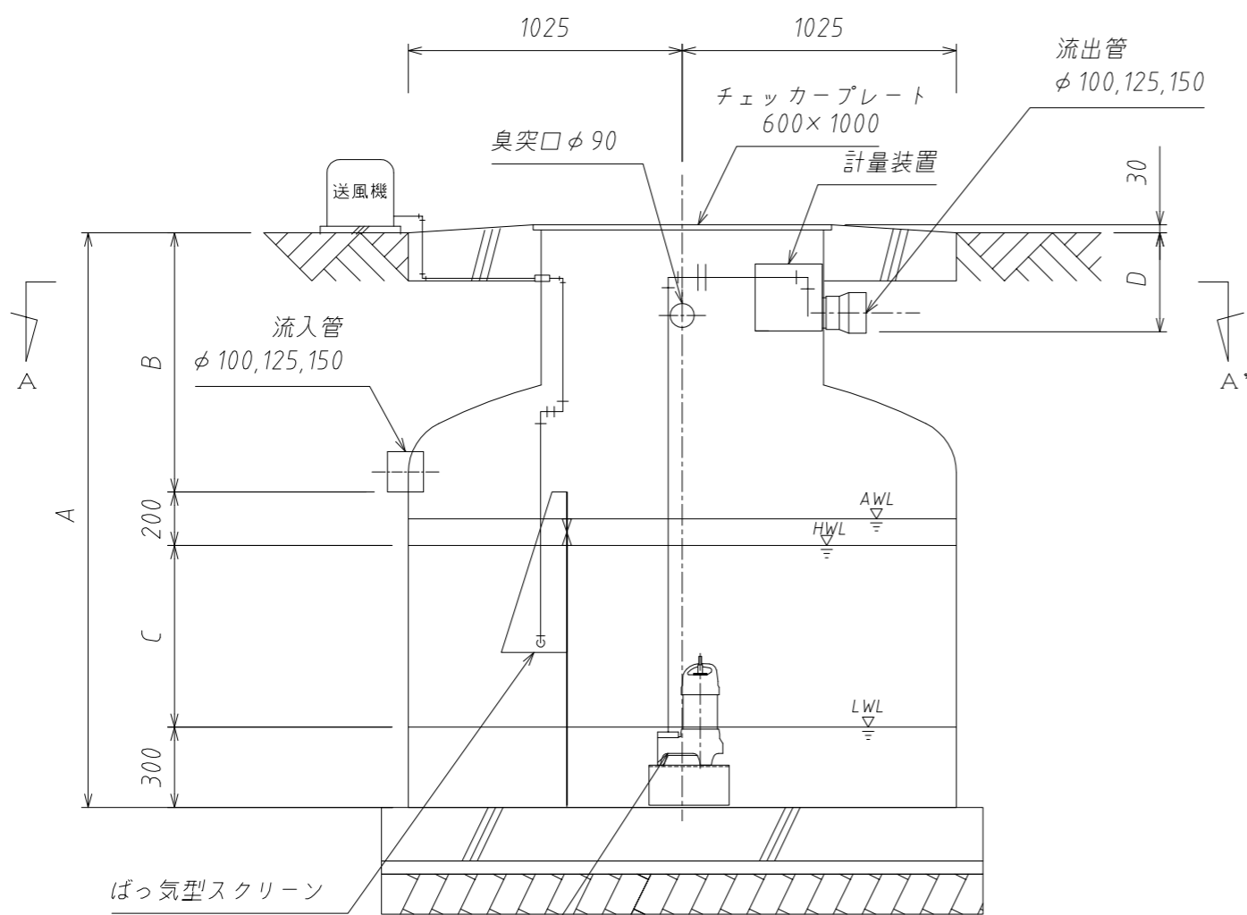
B-B' 断面図
