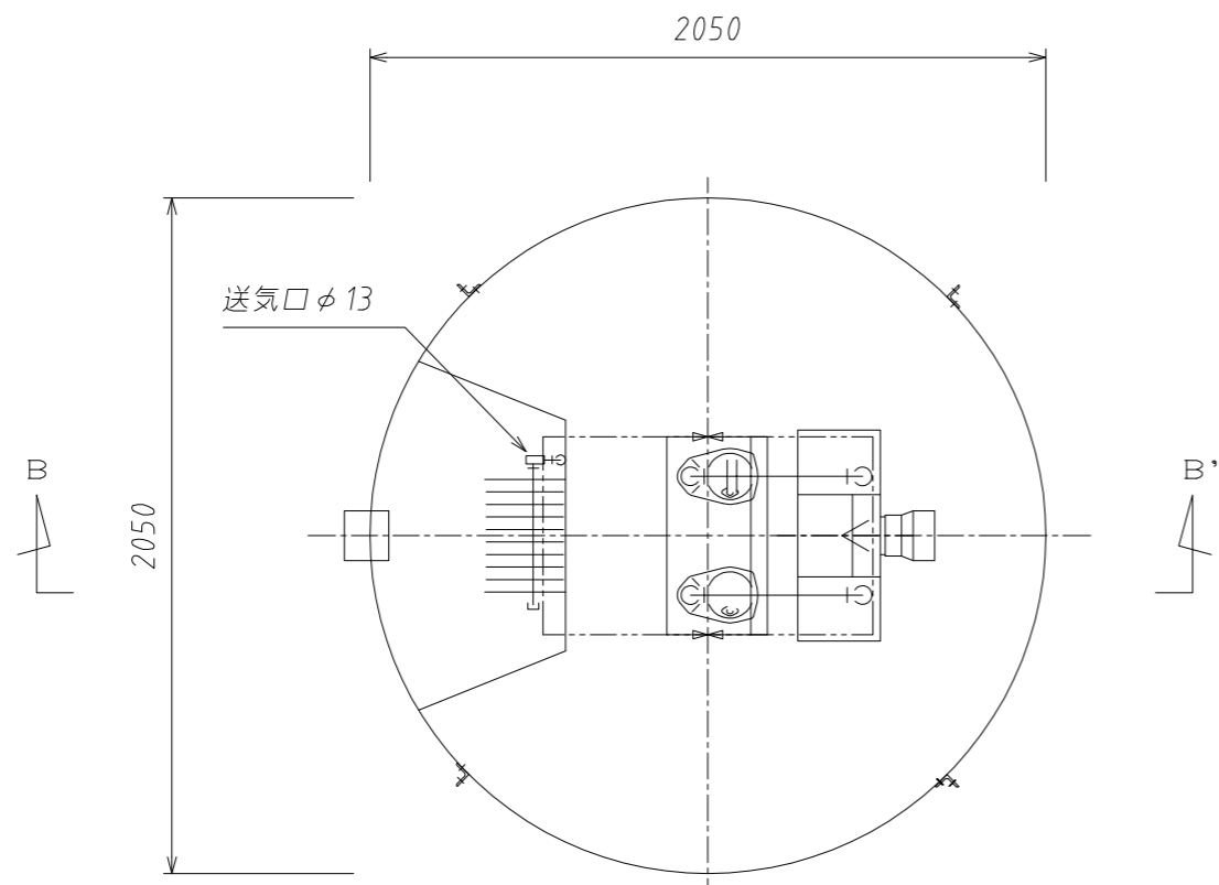
A-A' 断面図
