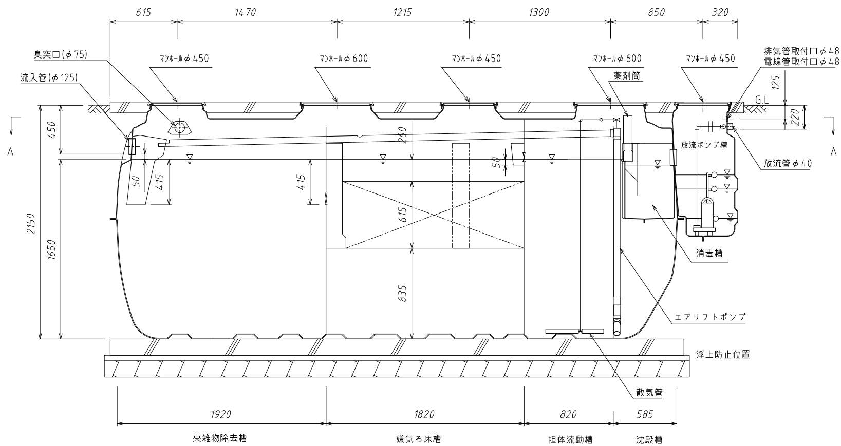
B-B断面図
