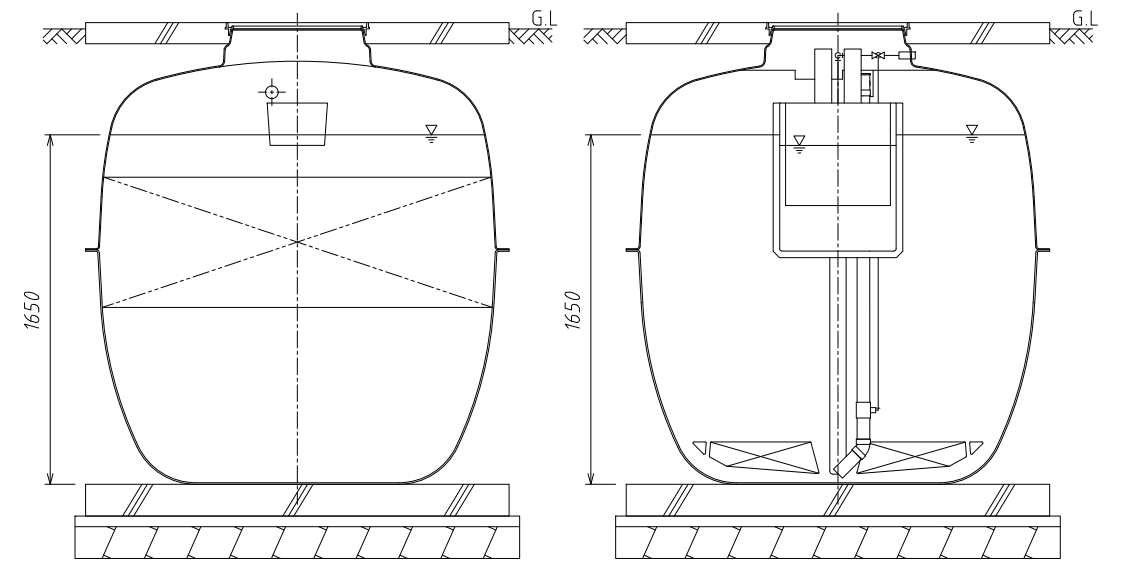
D-D断面図
