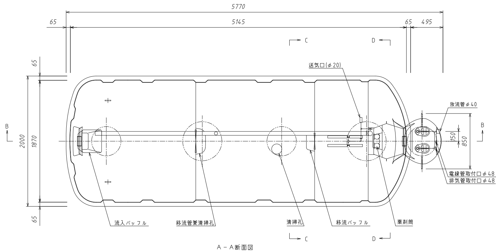
A-A断面図
