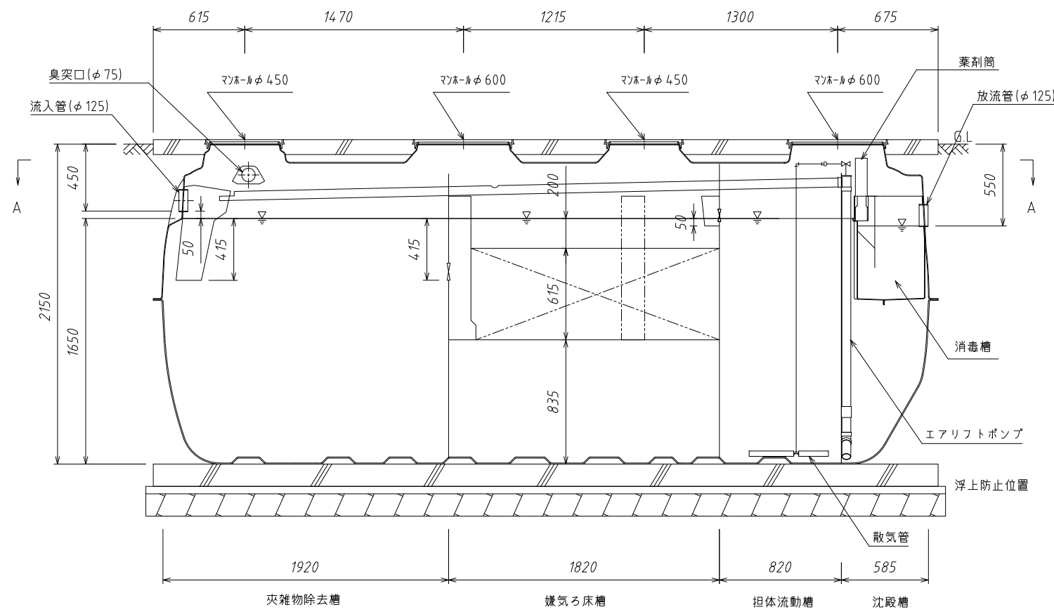
B-B断面図
