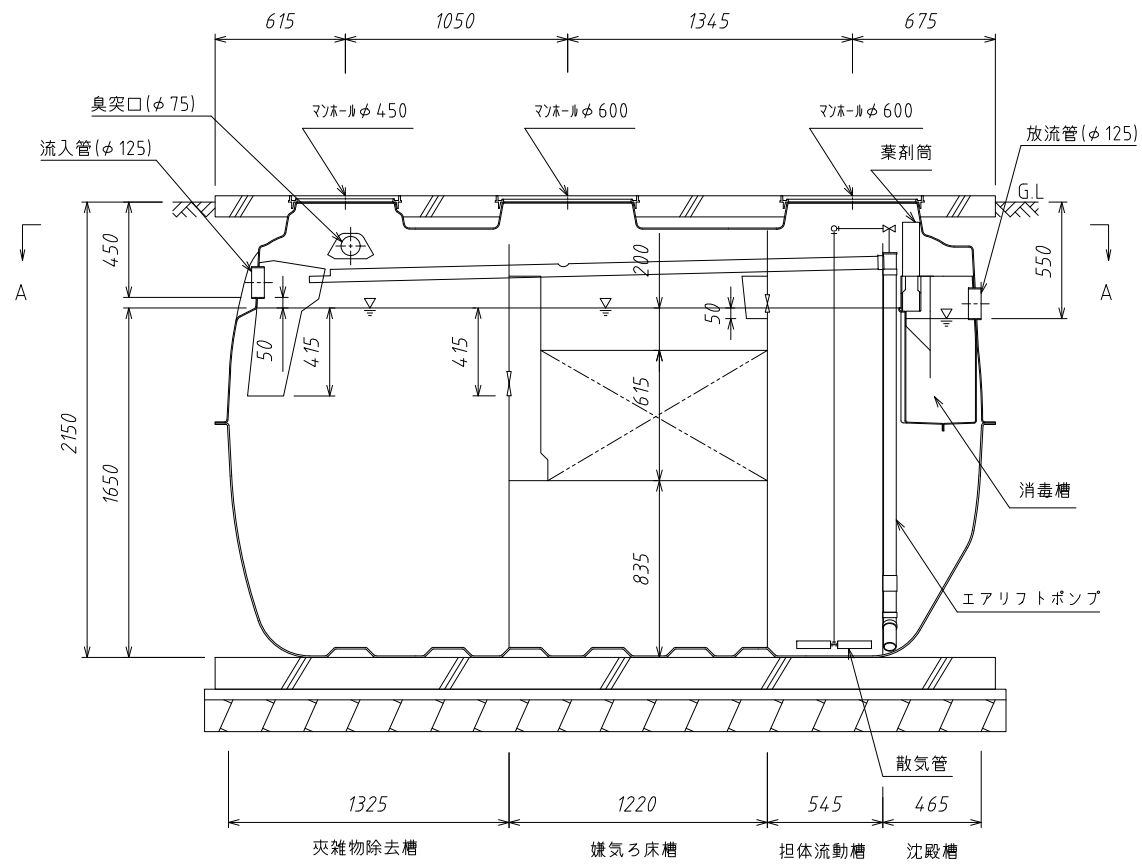
B-B断面図
