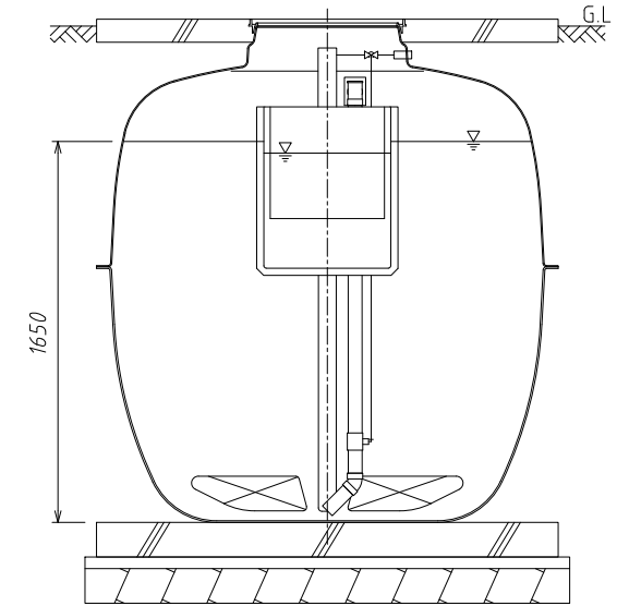
D-D断面図
