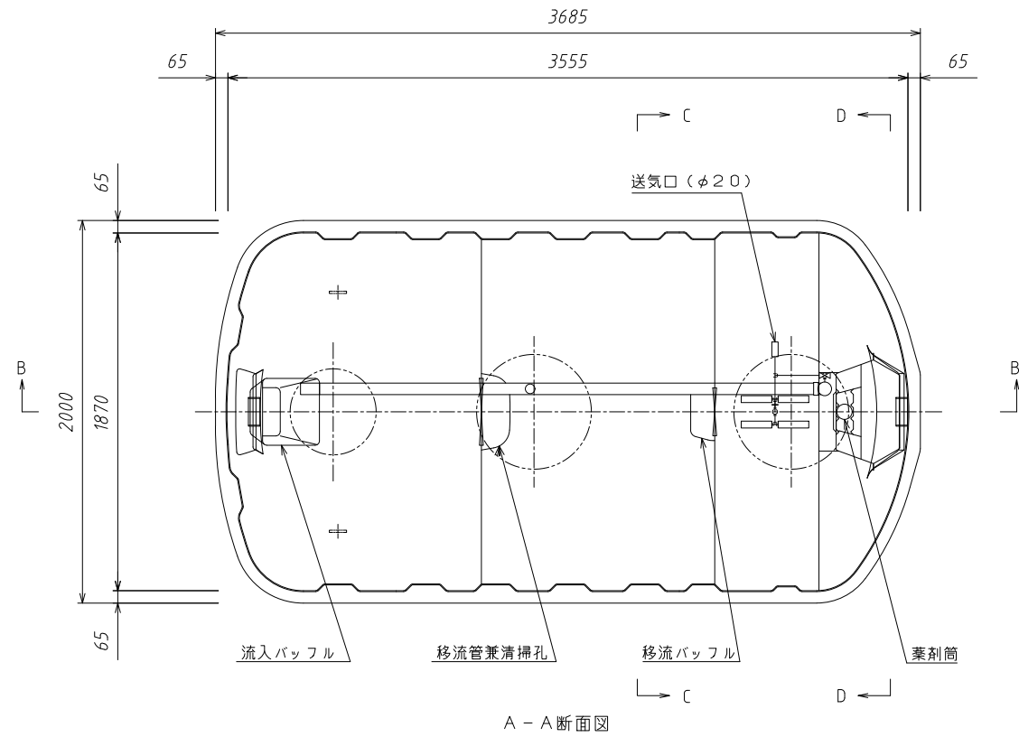
A-A断面図
