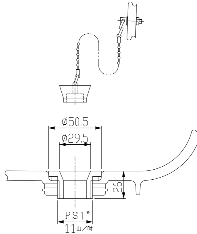
排水部詳細
