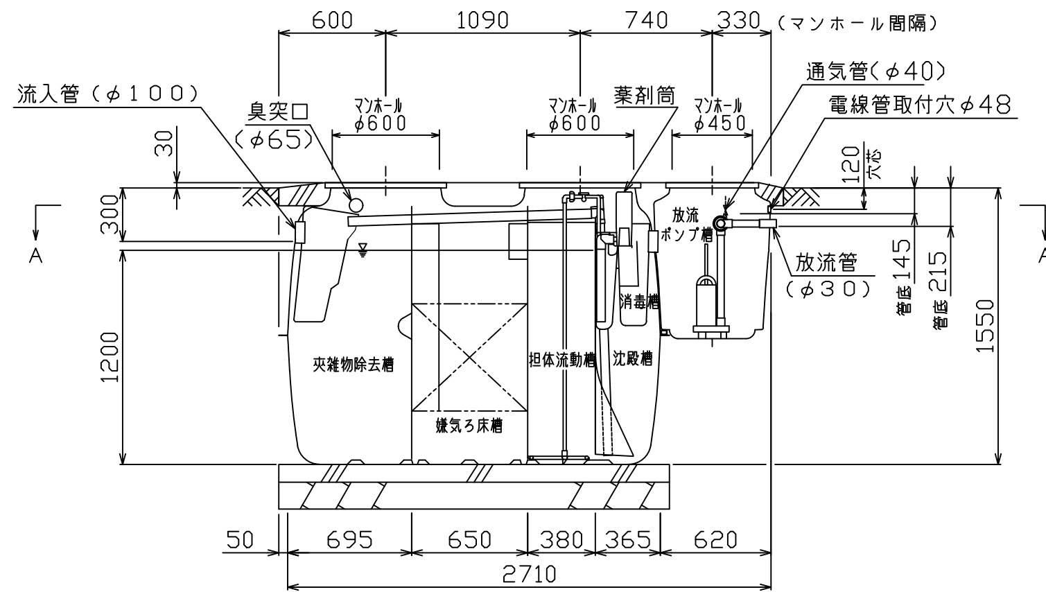
B-B断面図
