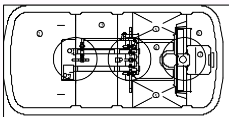
H Y型 構造概略図
