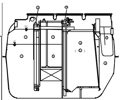
H Y型 構造概略図
