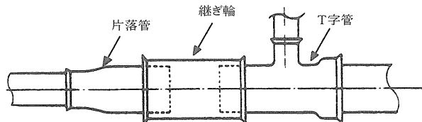
図 悪い配管例
