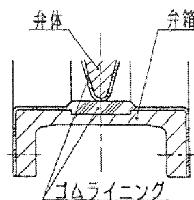
弁座部詳細
