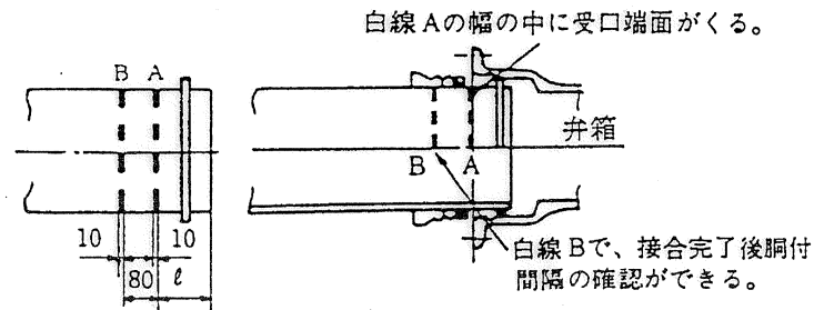
図-7 受口・挿し口の挿入完了
