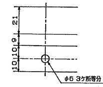
C 詳細図 S=1/2
