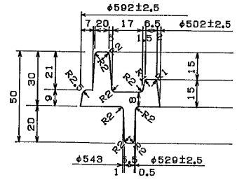
A-B 矢視 S=1/2
