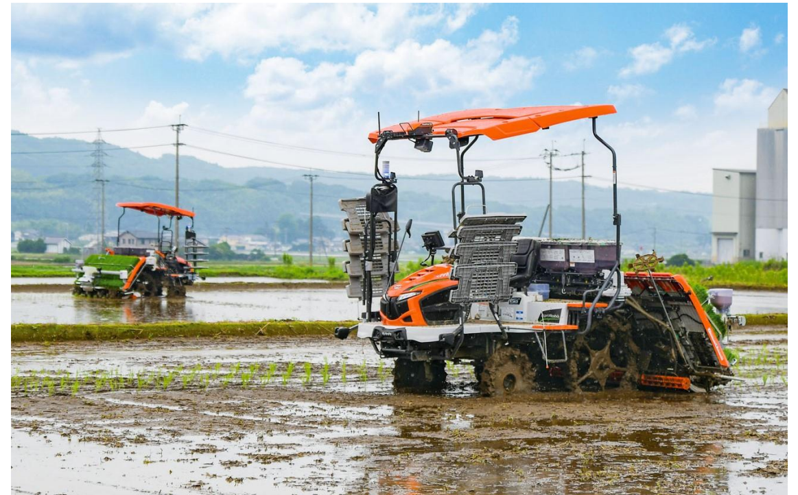
無人の自動運転田植機 2 台同時作業を実証
